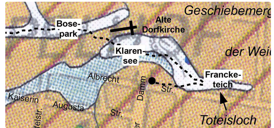
Ausschnitt: Alt-Tempelhof, geologische Karte von Berlin
